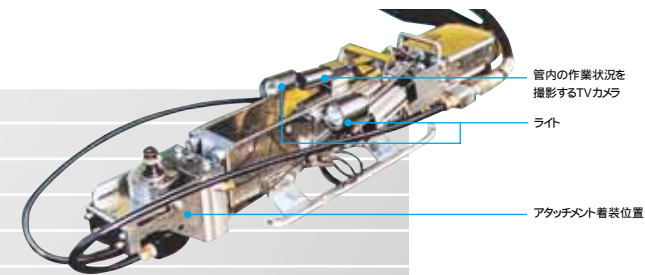
テレビモニターを見ながらICPロボットを操作。
